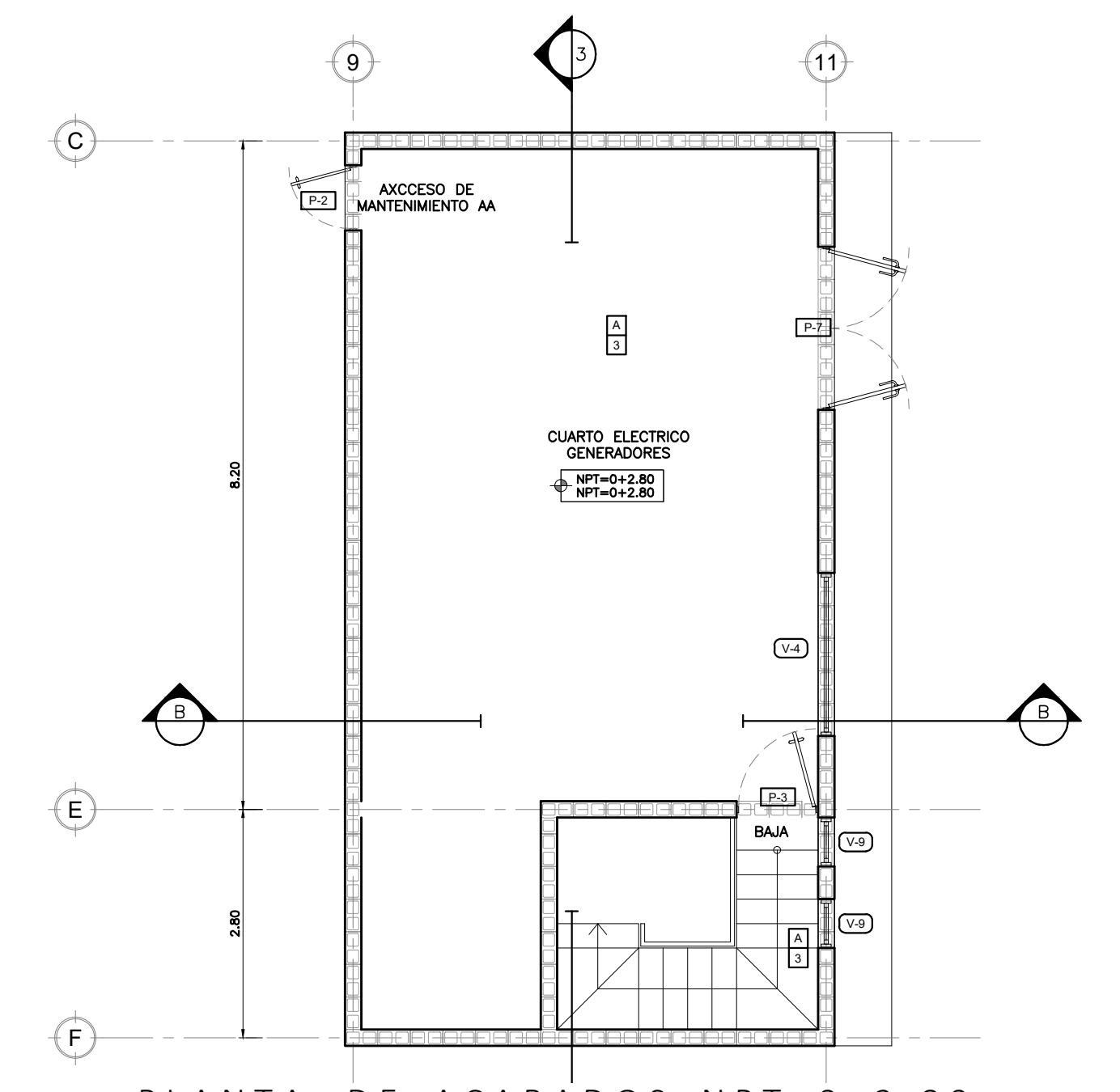
PLANTA DE ACABADOS NPT=0+2.80 REFORMULACION DE MODERNIZACION DE INSTALACIONES UEES HNZ ESC 1:75
