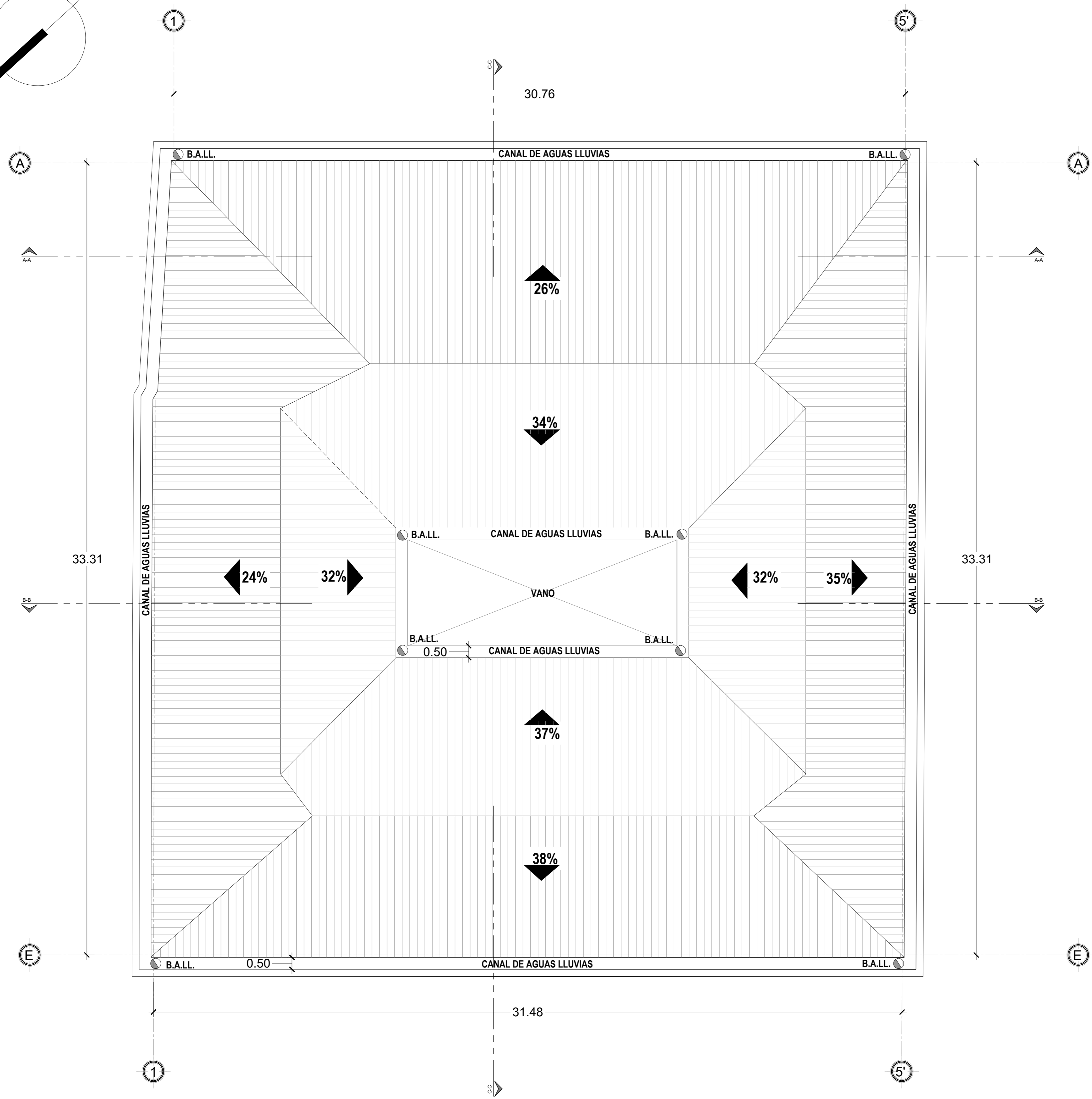
PLANTA ARQUITECTÓNICA DE TECHOS ESC.1:100
